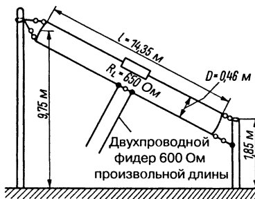
Рис. 10.42. Антенна T2FD согласно W3NH
