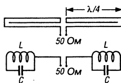
Рис. 10.29. Принцип действия двухдиапазонной антенны Mop-Gain в 40-метровом диапазоне
