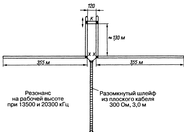
Рис. 18.6. Рефлектор направленной антенны G4ZU
