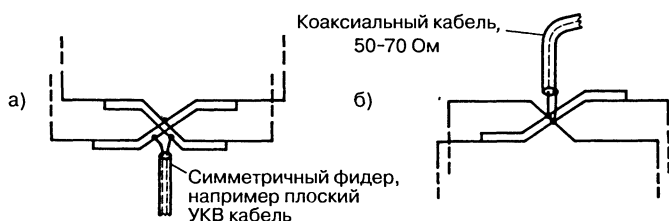
Рис. 15.18 Питание и возбуждение «швейцарского квадрата»: а – двоянное Т-образное согласование и питание; б – двоянное гамма-образное согласование и питание
