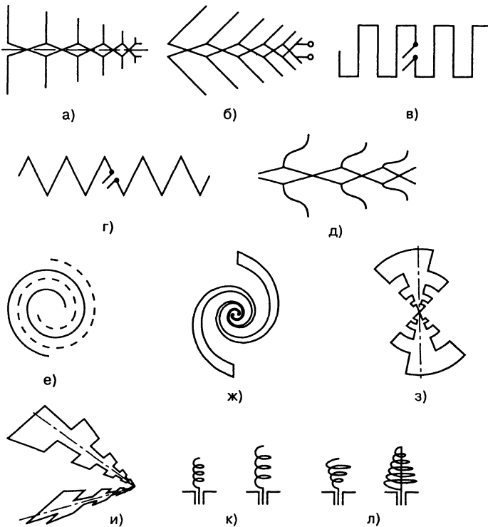
Рис. 4.3. Строение излучателей. Антенны: а – логопериодическая вибраторная; б – логопериодическая V-образная; в – в форме меандра; г – зигзагообразная; д – логопериодическая вибраторная по Ландсторферу; е – архимедова спираль; ж – логарифмическая спираль; з – логопериодическая планарная; и – логопериодические, соприкасающиеся передними концами; к – цилиндрическая спиральная; л – коническая спиральная
