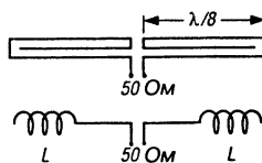
Рис. 10.28. Принцип действия двухдиапазонной антенны Mop-Gain в 80-метровом диапазоне
