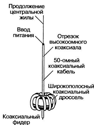
Рис. 7.51. Широкополосная коаксиальная катушка
