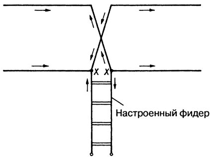
Рис. 13.13. Синфазная горизонтальная антенна с настроенным фидером
