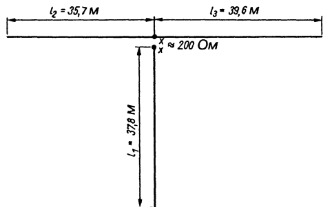
Рис. 11.23. Схема с размерами шестидиапазонной длиннопроводной антенны К4ЕF (вид сверху)
