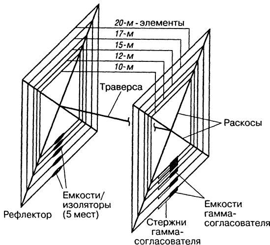
Рис 18.58 Пятидиапазонная двухэлементная рамочная антенна
