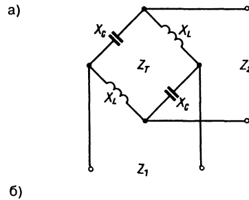
Рис. 6.24. Согласование с помощью моста Бушера: а – принципиальная схема; б – практический пример
