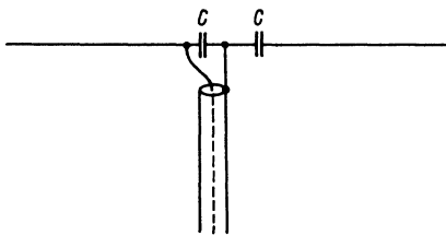
Рис. 7.76. Емкостный трансформатор
