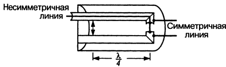
Рис. 7.37. V-образный симметрирующий трансформатор
