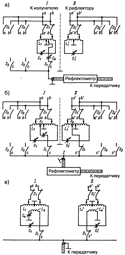
Рис. 18.31. Блок настройки многодиапазонной рамки DJ4VM: а – с пассивным рефлектором; б – со «сплошным» питанием; в – с индуктивной связью
