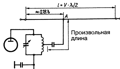
Рис. 10.10. Антенна Виндома
