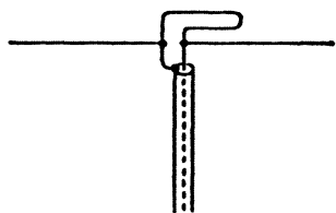
Рис. 7.75. L-согласование
