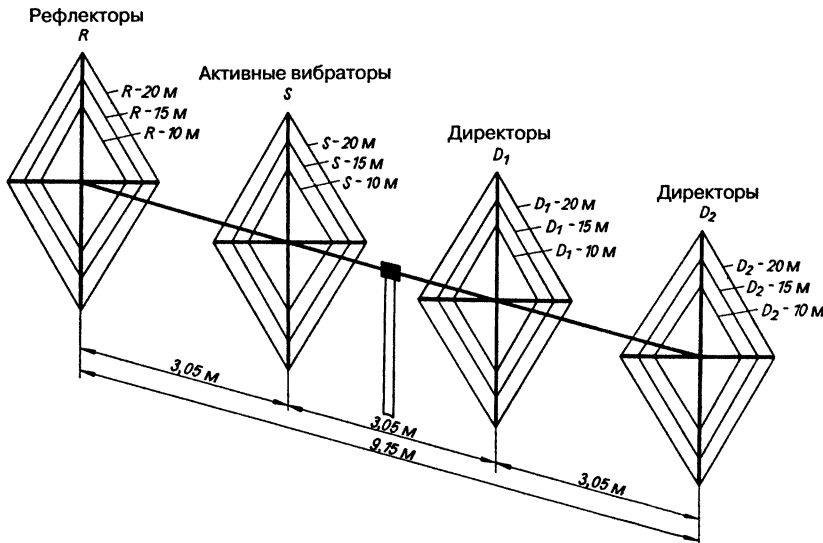
Рис. 18.56. Устройство и размеры четырехэлементной рамочной антенны
