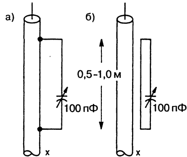
Рис. 7.44. Настроенный контур (блокирующие контуры на 14 МГц)
