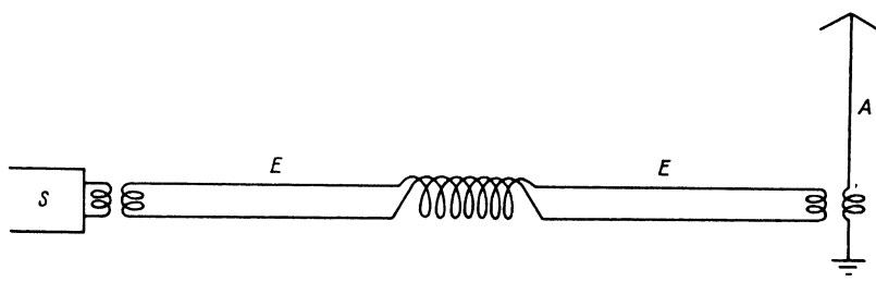
Рис. 7.48. Сифазный дроссель
