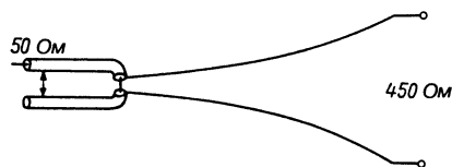
Рис. 7.31. Линия СТ
