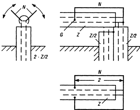
Рис. 7.27. Рамочный симметрирующий трансформатор
