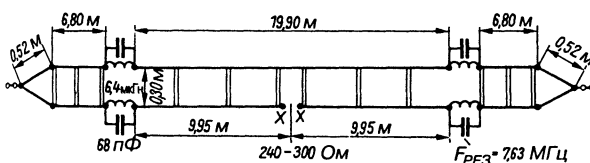
Рис. 10.25. Многодиапазонная антенна с запирающим контуром HA5DM
