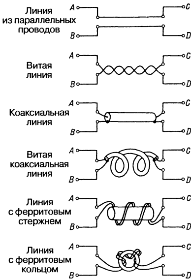
Рис. 7.7. Варианты исполнения линейных трансформаторов
