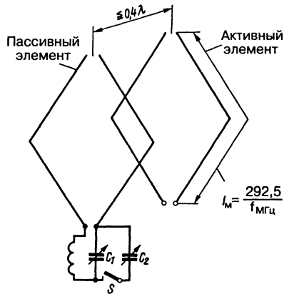
Рис. 13.19. Двойной двусторонний квадрат
