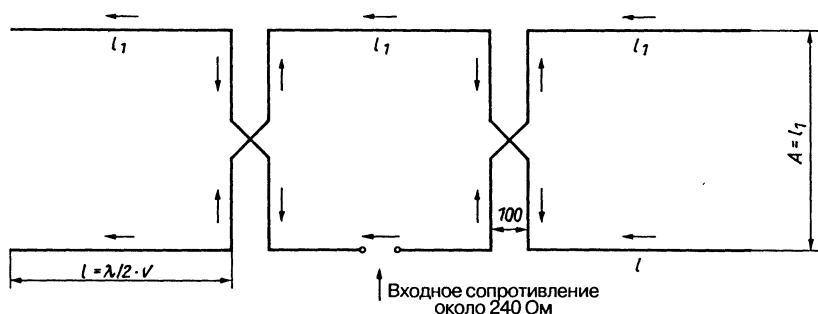
Рис. 13.21. Шестиэлементная антенна
