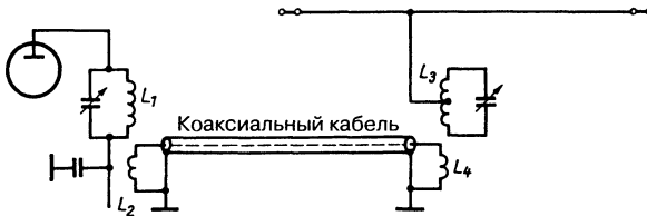
Рис. 10.13. Антенна Виндома с линией-связкой
