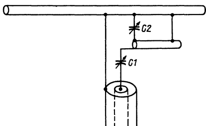
Рис. 7.74. Омега-согласование
