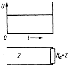
Рис. 5.21. Распределение напряжения в линии при согласовании
