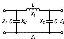
Рис. 6.26. П-образный согласующий элемент
