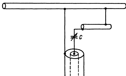
Рис. 7.73. Гамма-согласование
