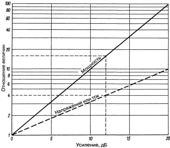
Рис. 3.17. Соотношения тока, напряжения и мощности для усиления
