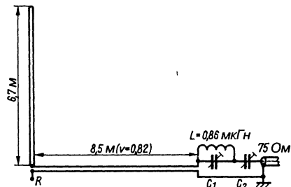
Рис. 19.55. Трехдиапазонная вертикальная антенна оператора OD5CG
