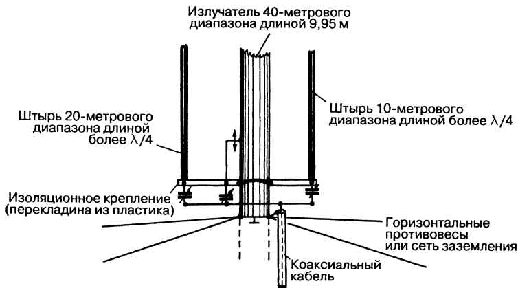
Рис. 19.57. Четырехдиапазонная Groundplane с кабельным согласованием
