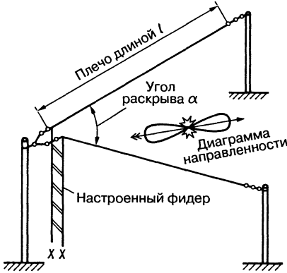
Рис. 11.12. Схема V-образного направленного излучателя
