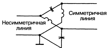
Рис. 7.33. Другая форма моста Бушера
