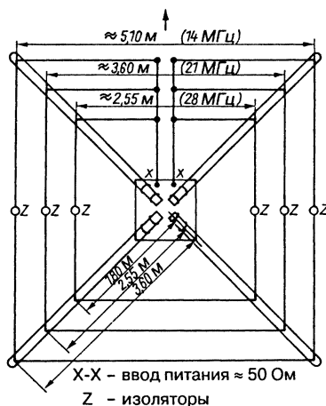
Рис. 18.42. Трехдиапазонная остронаправленная антенна VK2ABQ
