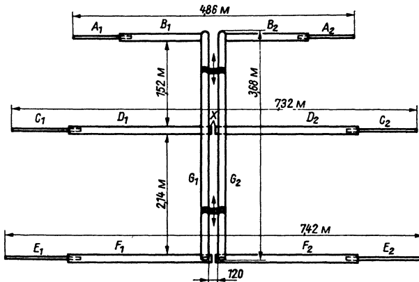
Рис. 18.8. Размеры проверенного образца антенны G4ZU
