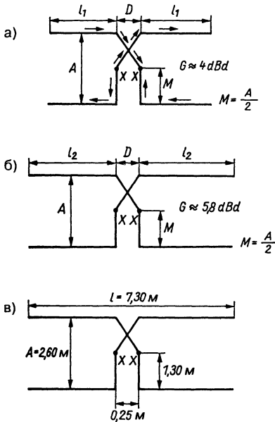
Рис. 14.5. Схема антенны W8JK: а – одна секция, соответствующая двум элементам; б – две секции, соответствующие четырем элементам; в – размеры для многодиапазонной работы, предложенные оператором W8JK
