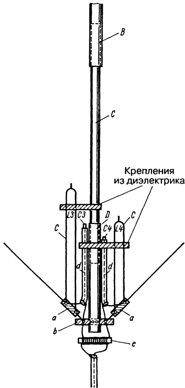
Рис. 18.29. Эскиз параллельного резонансного контура и ввода питания
