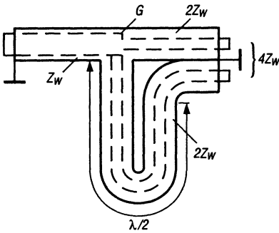
Рис. 7.12. Принцип действия полуволнового шлейфа
