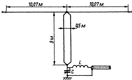
Рис. 19.54. Четырехдиапазонная антенна DL2EO
