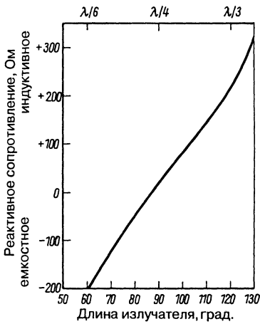
Рис. 19.46. Ориентировочные значения реактивного сопротивления вертикальной антенны над идеальным грунтом в зависимости от длины излучателя (1 λ соответствует 360°)
