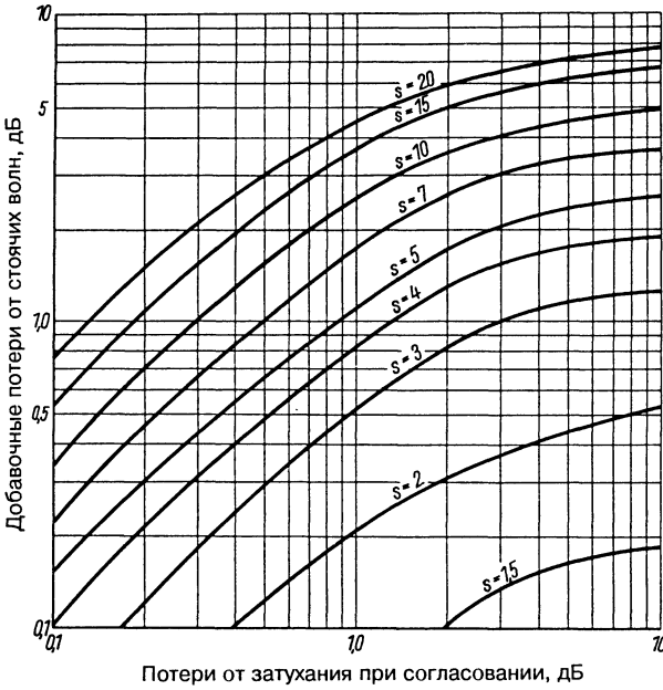
Рис. 5.25. Потери в линии, обусловленные рассогласованием
