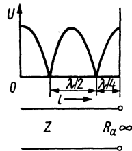
Рис. 5.22. Распределение напряжения в разомкнутой линии
