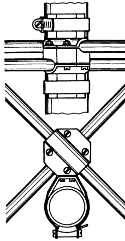
Рис. 15.21. Усовершенствованное крепление антенны к мачте
