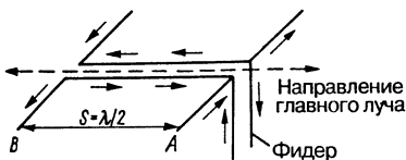
Рис. 14.1. Возбуждение и ток продольного излучателя
