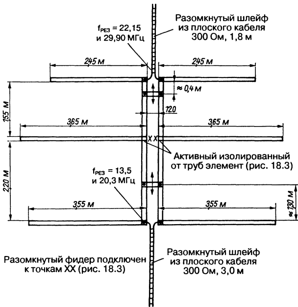
Рис. 18.7. Остронаправленная трехдиапазонная антенна G4ZU
