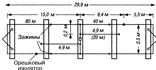
Рис. 10.31. Вложенная антенна для диапазонов 80, 40, 20 и 15 м
