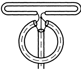
Рис. 7.13. Реализация полуволновой петли
