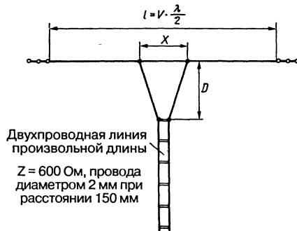
Рис. 10.1. Y-образная антенна
