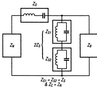
Рис. 7.40. Эквивалентная схема скомпенсированного симметрирующего трансформатора
