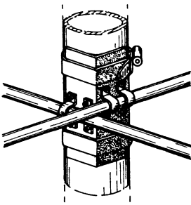
Рис. 15.20. Вариант простого крепления антенны к мачте
