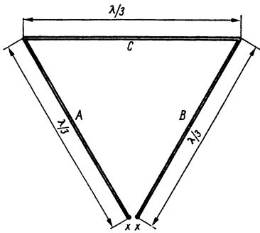
Рис. 15.6. Дельтообразная рамка
