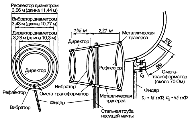
Рис. 15.14. Трехэлементная кольцевая антенна для 10-метрового диапазона
