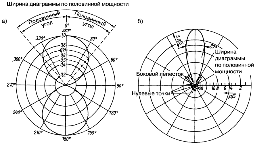
Рис. 3.8. Горизонтальные диаграммы направленности
