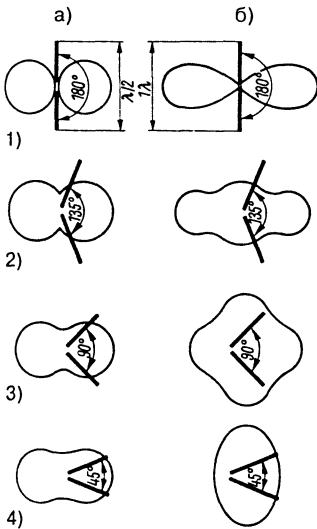
Рис. 10.36. Горизонтальные диаграммы направленности угловых вибраторов
