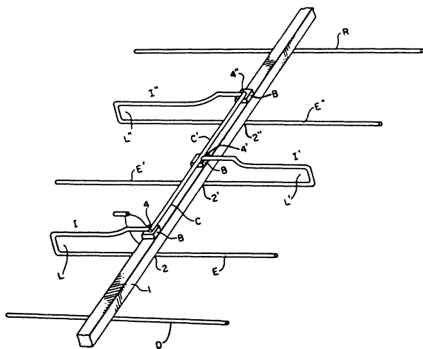
Рис. 7.72. Трансформатор на базе петлевого вибратора
