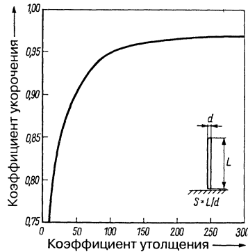
Рис. 19.8. Коэффициент укорочения V четвертьволнового штывра в зависимости от степени его утолщения
