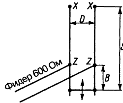
Рис. 14.6. Шлейф для антенны W8JK
