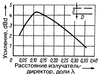
Рис. 16.2. Реальное усиление комбинации излучателя и пассивного директора
