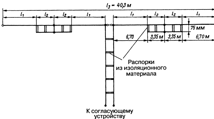
Рис. 13.11. Антенна JF
