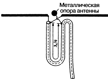
Рис. 7.47. Открытый блокирующий резонатор для диапазонов УКВ и ДМВ
