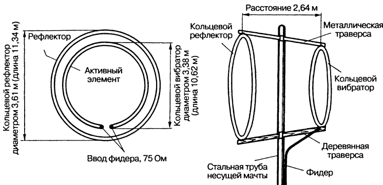
Рис. 15.13. Двухэлементная остронаправленная кольцевая антенна для 10-метрового диапазона
