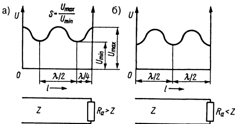
Рис. 5.24. Распределение напряжения в линии при рассогласовании
