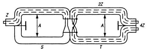
Рис. 7.26. Потенциал-трансформатор
