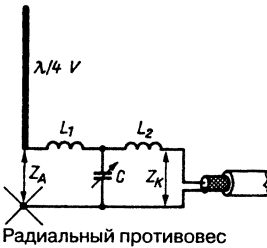
Рис. 19.14. Согласование антенны Groundplane через эквивалент трансформатора
