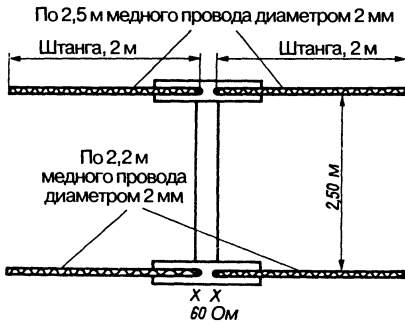
Рис. 17.7. Укороченный излучатель 10-метрового диапазона на удлинителях
