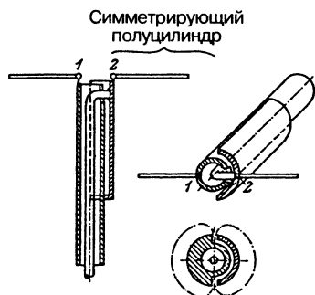
Рис. 7.30. Симметрирующий трансформатор с оболочкой-полуцилиндром
