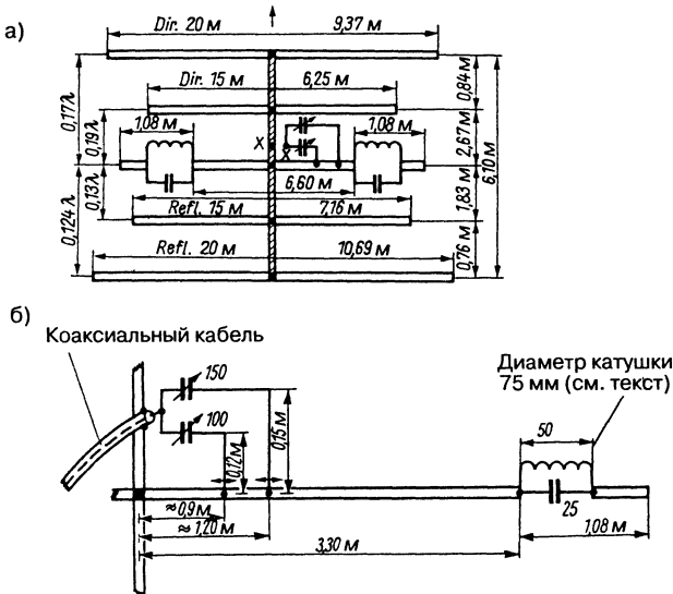
Рис. 18.37. Двухдиапазонная остронаправленная антенна КН6ОР на 20 и 15 м: а – общая схема; б – детализовка активного элемента
