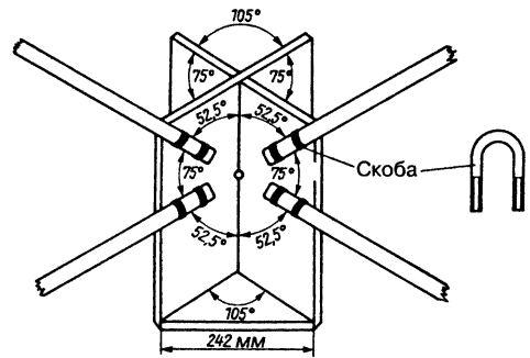
Рис. 18.50. Крепление кронштейнов
