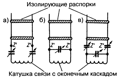
Рис. 5.36. Подключение фидера
