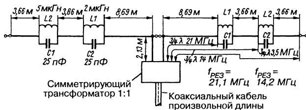
Рис. 10.27. Трехдиапазонная антенна W7QB (размеры указаны для резонансных частот 3, 7, 14,2 и 21,2 МГц)
