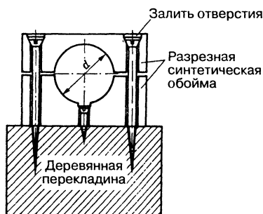
Рис. 17.4. Разрез блока для крепления элемента антенны
