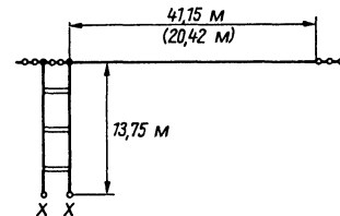
Рис. 10.7. Многодиапазонная антенна типа «Цеппелин»
