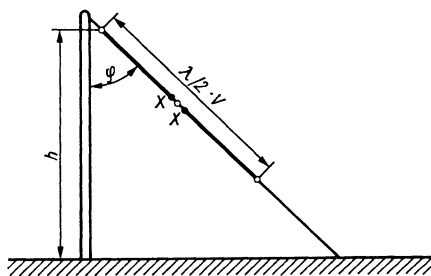
Рис. 10.38. Полуволновая наклонная антенна
