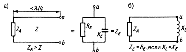
Рис. 6.12. Компенсация емкостной составляющей линии длиной меньше \lambda/4 : а – эквивалентная схема; б – компенсация X_E посредством X_L
