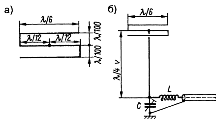
Рис 19.42 Оптимизированная Т-образная антенна а – схема сложной горизонтальной части, б – устройство антенны с Г-образным согласователем
