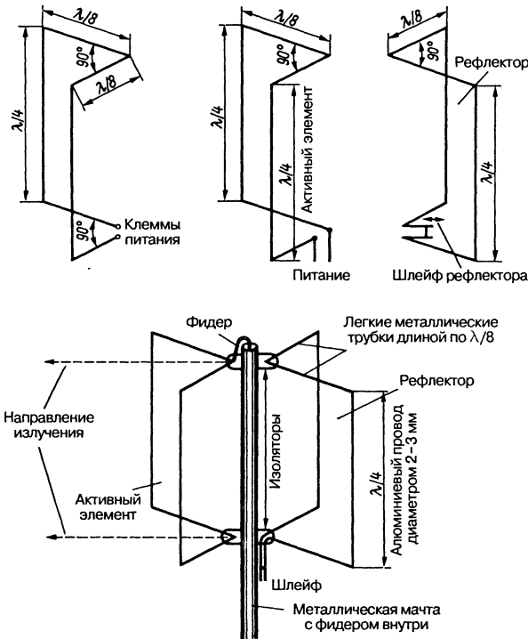
Рис. 15.15. Антенна G4ZU: а – квадратный элемент с изломом под 90°; б – схема антенны; в – вариант исполнения
