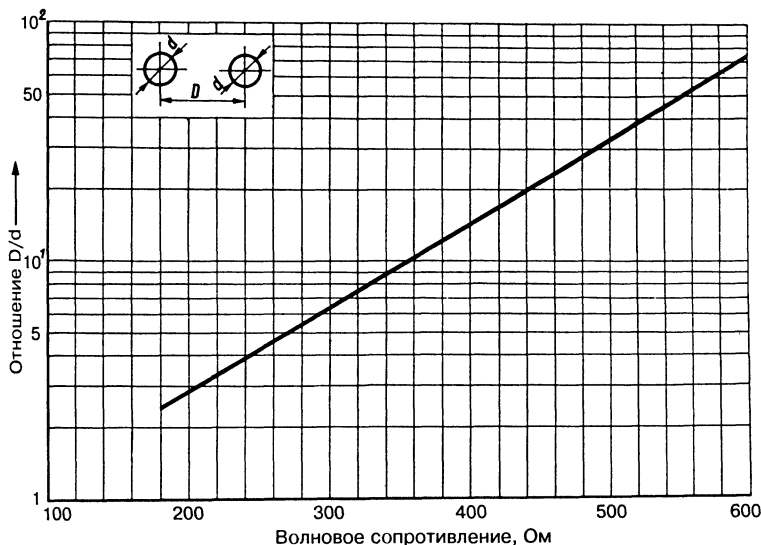
Рис. 5.4. Волновое сопротивление двухпроводной линии с воздушной изоляцией
