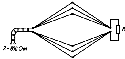
Рис. 12.12. Широкополосный ромб
