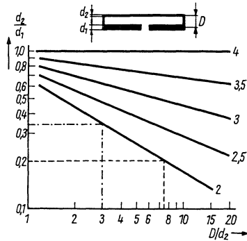
Рис. 19.23. Отношение входного сопротивления петлевого вибратора с неравными диаметрами элементов, приведенное к разному вибратору, в зависимости от d_2/d_1 и D/d_2
