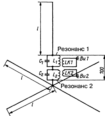
Рис. 19.62. Схема трехдиапазонной Groundplane с многодиапазонными контурами VK2AOU
