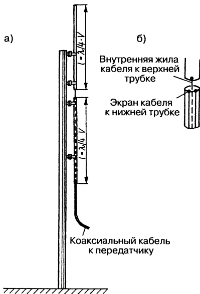
Рис. 19.34. Коаксиальная антенна: а – эскиз антенны; б – расписка ввода питания
