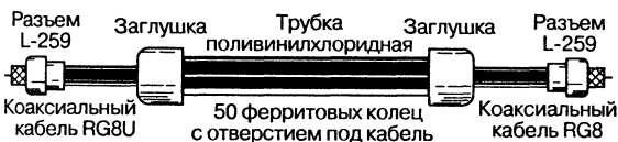
Рис. 7.57. Трансформатор W2DU
