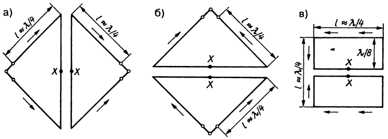
Рис. 13.16. Варианты рамки DJ4VM: а – ромбическая с горизонтальной поляризацией; б – то же с вертикальной поляризацией; в – квадратная с горизонтальной поляризацией
