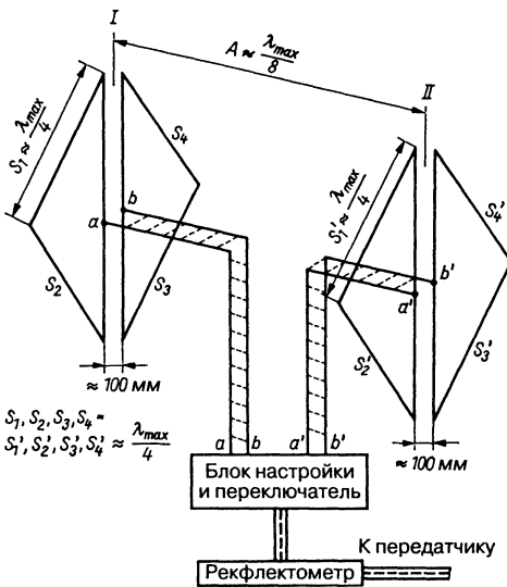
Рис. 18.30. Эскиз многодиапазонной рамки DJ4VM
