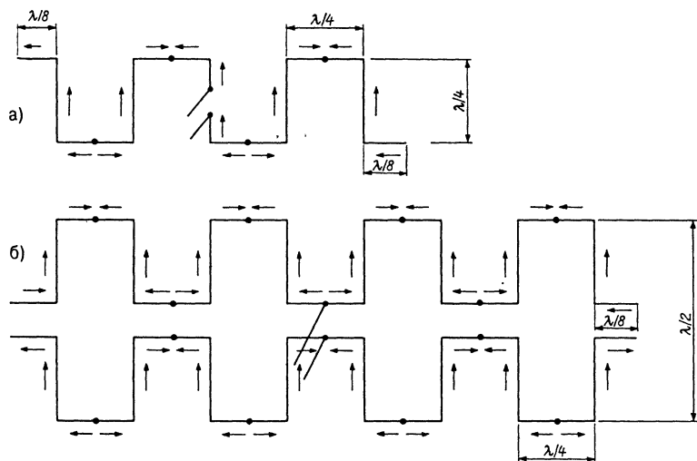
Рис. 13.22. Антенны Брюса: а – простая, б – сдвоенная
