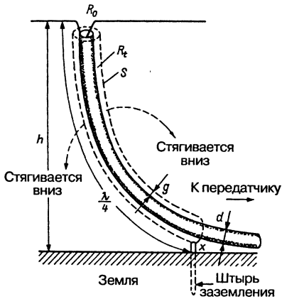
Рис. 7.46. Высокочастотный открытый коаксиальный трансформатор
