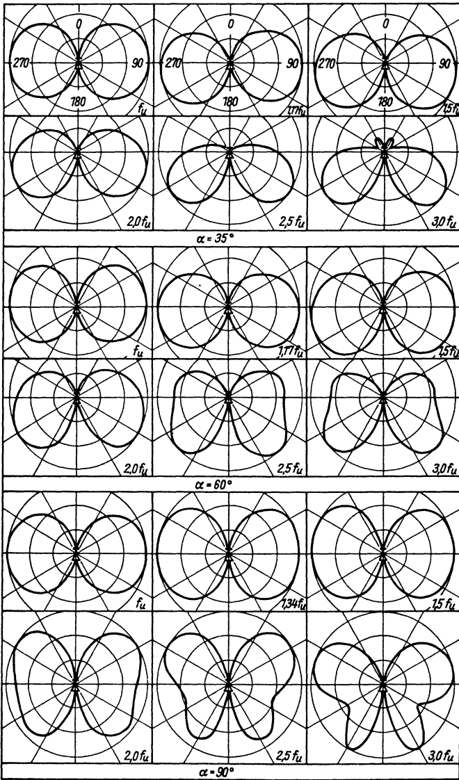
Рис. 19.72. Нормированные диаграммы направленности в плоскости E для дисконусных антенн с углом раскрыва \alpha 35°, 60° и 90° (по Нейлу)
