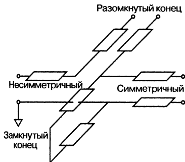
Рис. 7.38. Принципиальная схема скомпенсированного симметрирующего трансформатора
