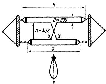
Рис. 14.9. Однонаправленная антенна ZL
