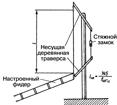
Рис. 19.35. Вертикальный полуволновый излучатель с питанием типа «Цепелин»
