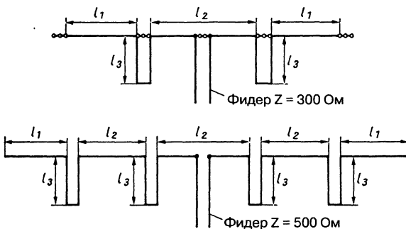
Рис. 13.10. Антенна Франклина: а – три коллинеарных вибратора, усиление 3,2 dB; б – пять коллинеарных вибраторов, усиление 5,2 dB
