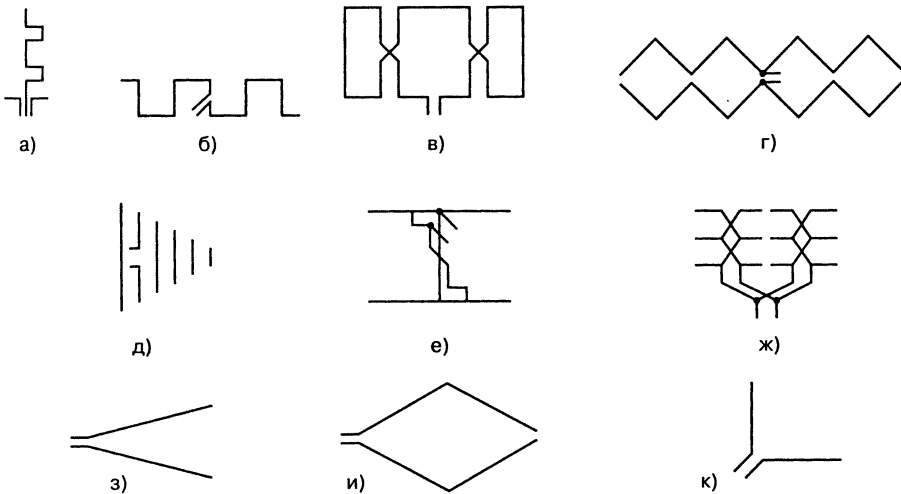
Рис. 4.2. Групповые излучатели – антенны: а – Франклина; б – Брюса; в – Стербы; г – Ширэ-Мезини; д – Уда-Яги («волновой канал»); е – NV9CV; ж – полотно вибраторов; з – V-образная; и – ромбическая; к – квадратная
