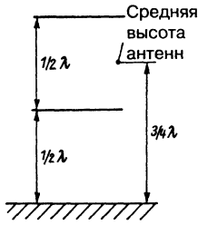
Рис. 3.14. Пример определения эффективной высоты многоэтажной горизонтальной антенны над идеальным грунтом
