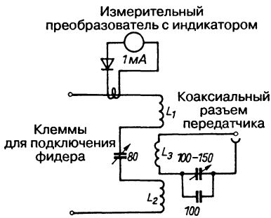
Рис. 18.11. Схема настроечного блока для антенны G4ZU: L_1 и L_2 – по 4 витка медного провода диаметром 1,5 мм, L_3 – 3 витка того же провода; бескаркасные катушки с диаметром намотки 40 мм
