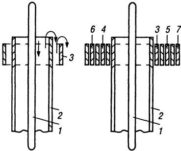
Рис. 7.56. Устройство поглотителя
