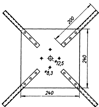
Рис. 18.54. Пластина с несущей крестовиной
