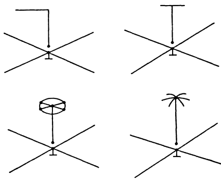
Рис. 19.30. Популярные типы вертикальных антенн с концевыми емкостями
