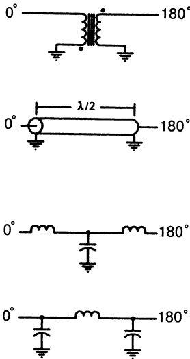
Рис. 7.4. Способы получения фазового сдвига на 180°
