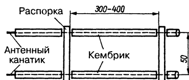
Рис. 18.19. Фидер
