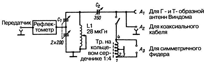
Рис. 8.15. Базовый СЛП
