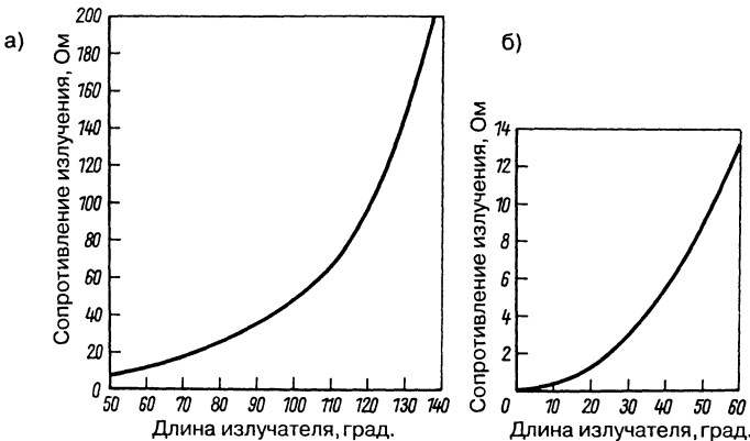
Рис. 19.47. Сопротивление излучения вертикальной антенны над идеальным грунтом в зависимости от длины излучателя: а – для длин излучателя между 50° и 140°; б – для длин менее 60°
