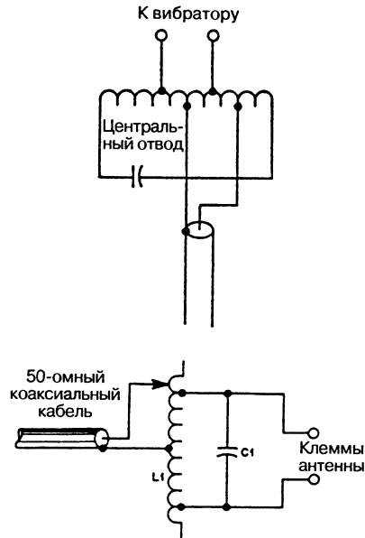
Рис. 7.6. Резонансный согласующий трансформатор с LC-цепочкой
