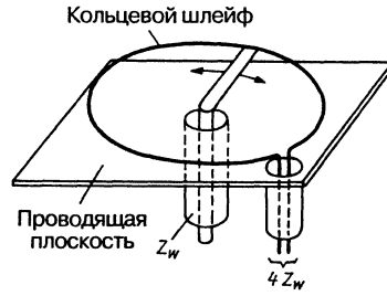
Рис. 7.17. Фазовый трансформатор
