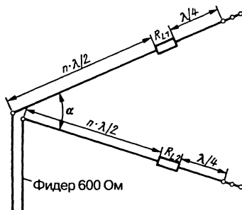
Рис. 12.7. Замкнутая V-образная антенна
