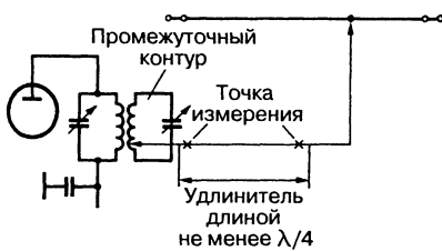
Рис. 10.11. Антенна Виндома с промежуточным контуром и отрезком-удлинителем
