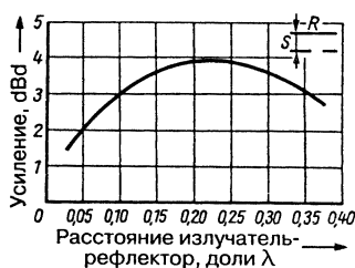
Рис. 16.1. Реальное усиление комбинации излучателя и пассивного рефлектора
