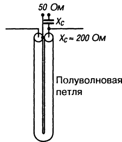
Рис. 10.45. Удлиненный вибратор
