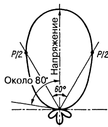
Рис. 15.19. Диаграмма направленности антенны «швейцарский квадрат»
