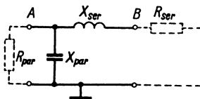
Рис. 19.49. Трансформатор реактивностей
