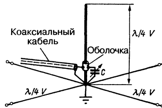
Рис 19.16 Заземленная антенна Groundplane
