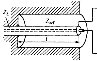
Рис. 7.41. Схема четвертьволнового блокирующего резонатора
