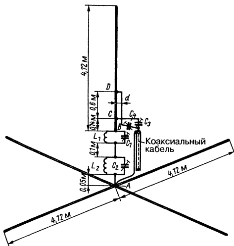
Рис. 19.58. Устройство трехдиапазонной Groundplane с многодиапазонными контурами
