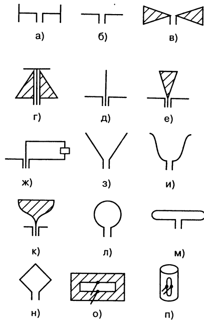
Рис. 4.1. Простые излучатели: а – вибратор Герца; б – вибратор; в – конический вибратор; г – дисконусная антенна; д – монополь; е – коническая антенна; ж – однопроволочная антенна бегущей волны (антенна Бевереджа); з – уголкоый вибратор; и – антенна «взмах крыла»; к – чашечный излучатель; л – петлевая антенна; м – петлевой вибратор; н – квадратная рамочная антенна; о – шелевая антенна; п – трубчато-шелевая антенна
