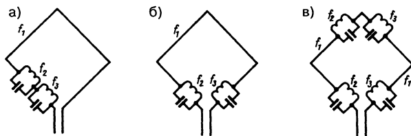
Рис. 18.27. Схема трехдиапазонного рамочного элемента, предложенного VK2AOU: а – конфигурация, соответствующая рис. 18.26а; б – симметричное включение f_2 и f_3 относительно входа антенны; в – парное расположение f_2 и f_3
