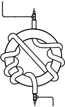
Рис. 7.52. Дроссель поверхностных волн
