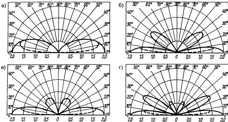
Рис. 3.16. Вертикальная диаграмма вертикального полуволнового вибратора
