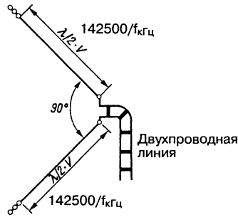
Рис. 10.37. Волновый угловой вибратор с круговой диаграммой направленности
