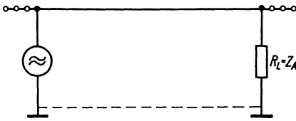
Рис. 12.1. Аперриодическая антенна
