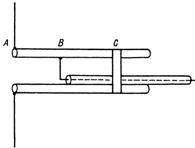
Рис. 7.22. Шлейф Пози
