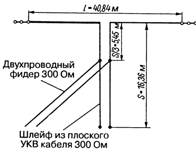
Рис. 10.19. Четырехдиапазонный вибратор
