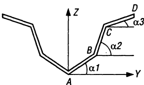
Рис. 10.44. Оптимизированный вибратор (ломаная из трех отрезков)
