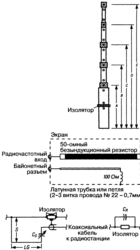
Рис. 18.59. Отдельные узлы антенны
