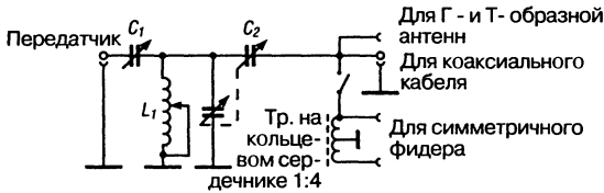
Рис. 8.17. СЛП на последовательно-параллельных емкостях
