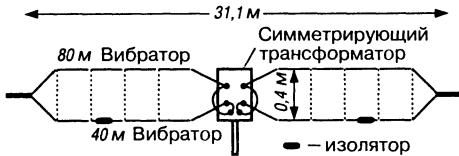
Рис. 10.30. Укороченная трехдиапазонная антенна для диапазонов 80, 40 и 15 м
