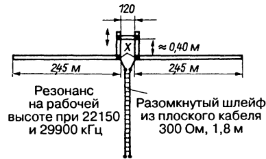
Рис. 18.5. Директор направленной антенны G4ZU
