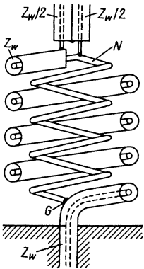
Рис. 7.23. Устройство широкополосного симметрирующего шлейфа
