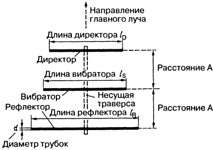
Рис. 16.10. Схема трехэлементной директорной антенны
