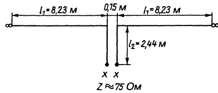
Рис. 11.22. Двухдиапазонный вариант антенны ГЗТКН (указаны размеры для 7 и 21 МГц)
