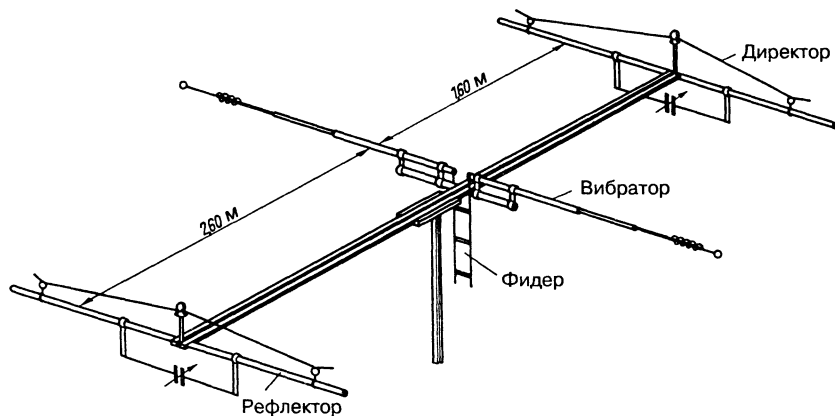
Рис. 18.22. Антенна DL1FK
