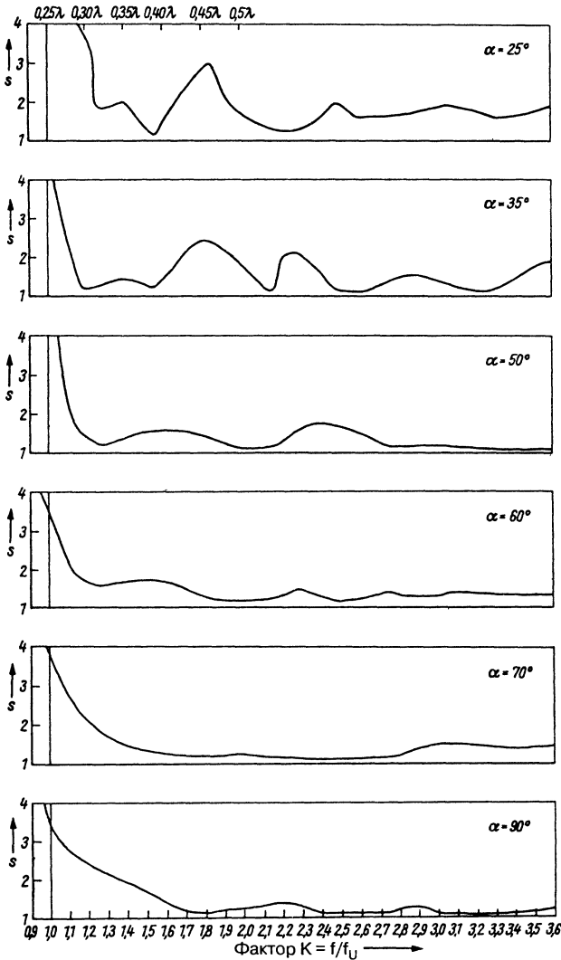
Рис. 19.71. Согласование дисконусной антенны и 50-омного коаксиального кабеля при различных углах раскрытия \alpha в зависимости от рабочей частоты
