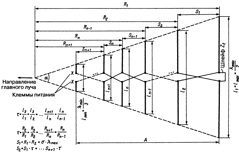
Рис. 18.66. Схема и размеры логопериодической вибраторной антенны
