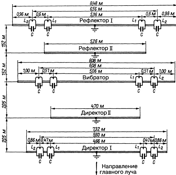
Рис. 18.24. Схема остронаправленной трехдиапазонной антенны W3DZZ
