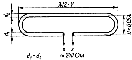
Рис. 3.21. Петлевой вибратор
