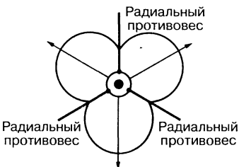
Рис. 19.19. Горизонтальная диаграмма направленности антенны с тремя противовесами
