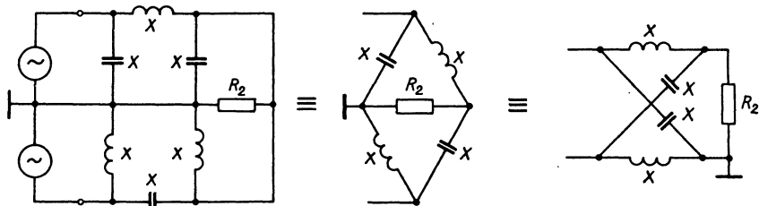
Рис. 7.32. Формирование моста Бушера
