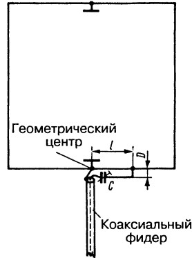
Рис. 15.12. Активный элемент рамочной антенны с гамма-образным согласованием
