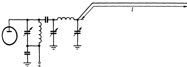
Рис. 11.6. Подключение Г-образной антенны через П-образный фильтр
