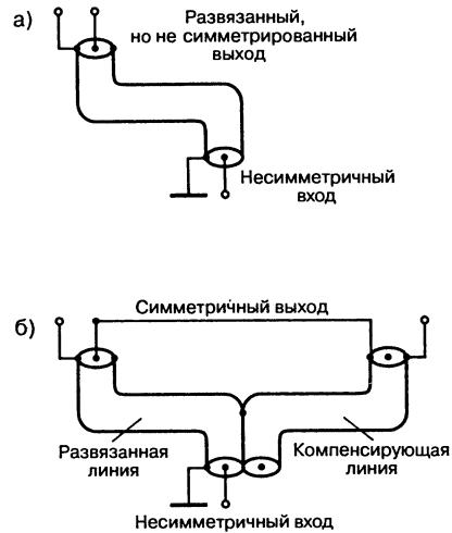
Рис. 7.9. Симметрирующий трансформатор: а – одиночный развязанный линейный трансформатор; б – он же после симметрирования посредством компенсирующей линии
