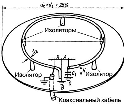
Рис. 19.64. Схема антенны DDRR
