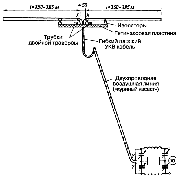
Рис. 18.3. Активный элемент направленного поворотного излучателя G4ZU
