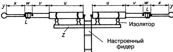
Рис. 18.18. Активный элемент антенны DL1FK
