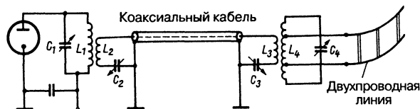
Рис. 8.8. Схема подключения произвольных согласованных симметричных линий передачи
