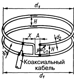
Рис. 19.65. Эскиз модифицированной антенны DDRR (изоляторы-распорки не показаны)
