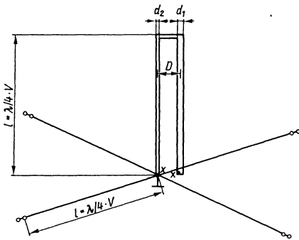
Рис. 19.22. Антенна Groundplane с двумя проводниками разного диаметра
