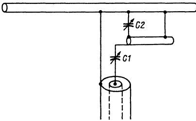
Рис. 6.5. Принцип действия омега-трансформатора
