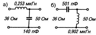
Рис. 6.22. Г-образный согласующий элемент
