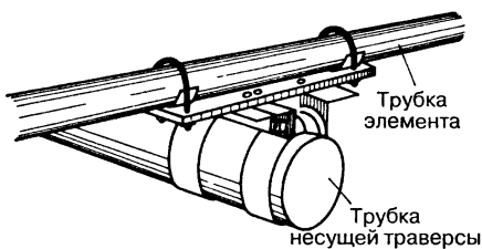
Рис. 16.11. Вариант крепления трубчатого элемента к траверсе антенны
