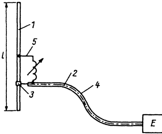
Рис. 7.70. Полуволновый барьер
