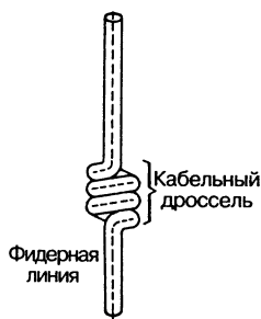
Рис. 7.49. Кабельный дроссель
