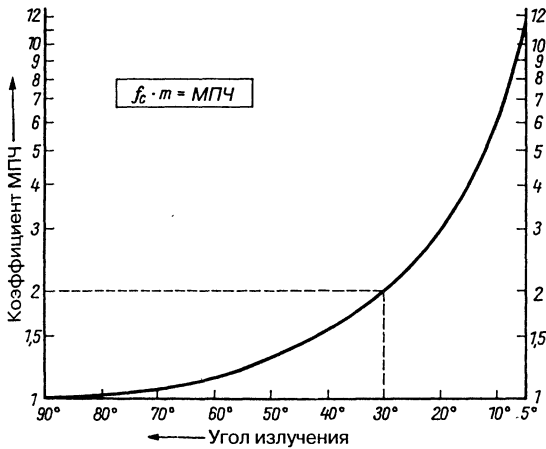
Рис. 2.6. Зависимость коэффициента МПЧ от угла излучения
