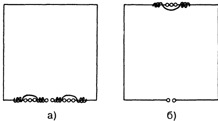
Рис. 15.4. Проволочные перемычки как средство подстройки рамочного элемента
