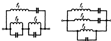
Рис. 18.26. Трехдиапазонный резонансный контур в двух вариантах
