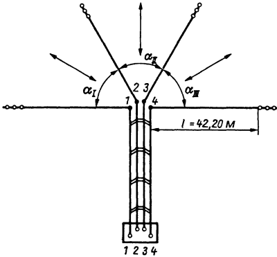
Рис. 11.15. Упрощенная звезда из V-образных излучателей
