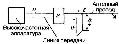
Рис. 7.18. Шлейф Картера
