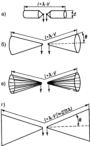
Рис. 10.40. Широкополосные вибраторы: а – «толстый» волновой вибратор из цилиндрических стержней, сведенных на конус; б – двухконусный вибратор; в – волновой вибратор с двумя коническими «корзинами»; г – плоский вибратор
