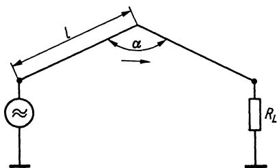
Рис. 12.6. Замкнутая тупоугольная V-образная антенна
