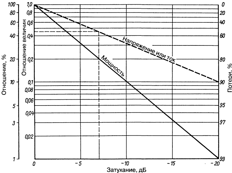
Рис. 3.18. Соотношения тока, напряжения и мощности для затухания
