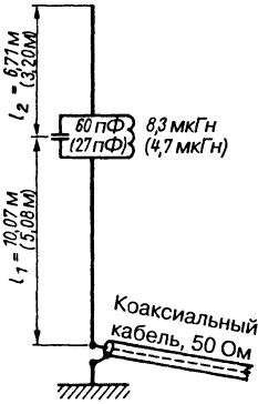
Рис. 19.61. Вертикальная антенна с контурами-ловушками для диапазонов 80 и 40 м
