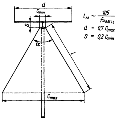
Рис. 19.69. Принципиальная схема дисконусной антенны
