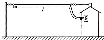
Рис. 11.4. Г-образная антенна
