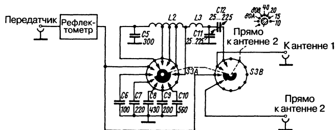
Рис. 8.18. П-образный фильтр (фильтр Коллинза)
