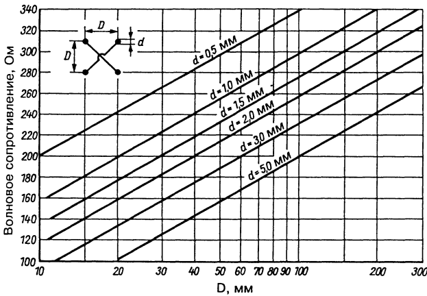
Рис. 5.15. Волновое сопротивление четырехпроводного фидера
