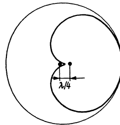
Рис. 14.8. Диаграмма направленности в виде кардиоиды
