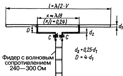
Рис. 6.3. Емкостные компенсаторы в согласующем Т-элементе
