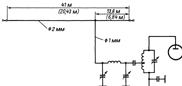
Рис. 10.14. Многодиапазонная антенна Виндома версии VS1AA
