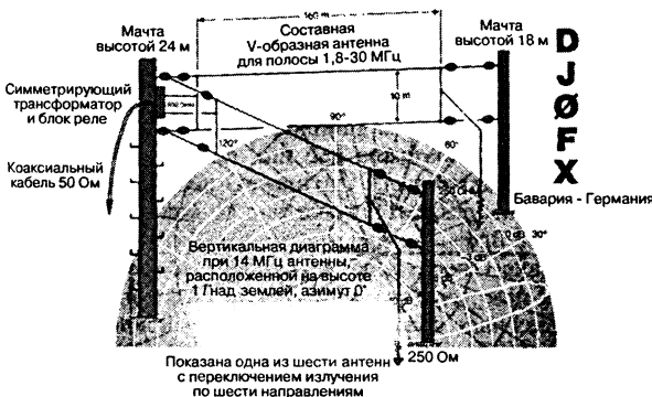
Рис. 11.16. Составная V-образная антенна
