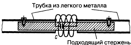
Рис. 18.25. Вариант исполнения запирающего контура
