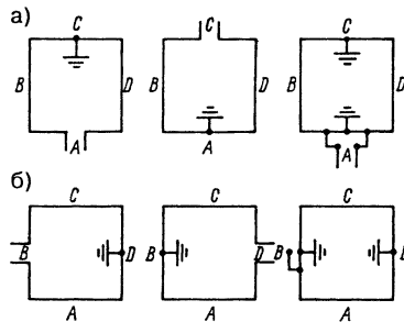
Рис. 15.3. Поляризация и возможности заземления квадратной рамки:
