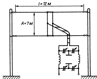
Рис. 13.15. «Ленивая Н» для работы в трех диапазонах
