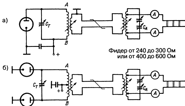
Рис. 8.7. Усовершенствованное подключение ненастроенной симметричной двухпроводной линии: а – однокатный, б – двухкатный оконечные каскады
