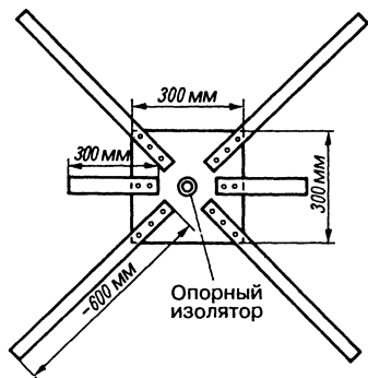
Рис. 19.59. Вариант деревянного опорного узла для трехдиапазонной Groundplane
