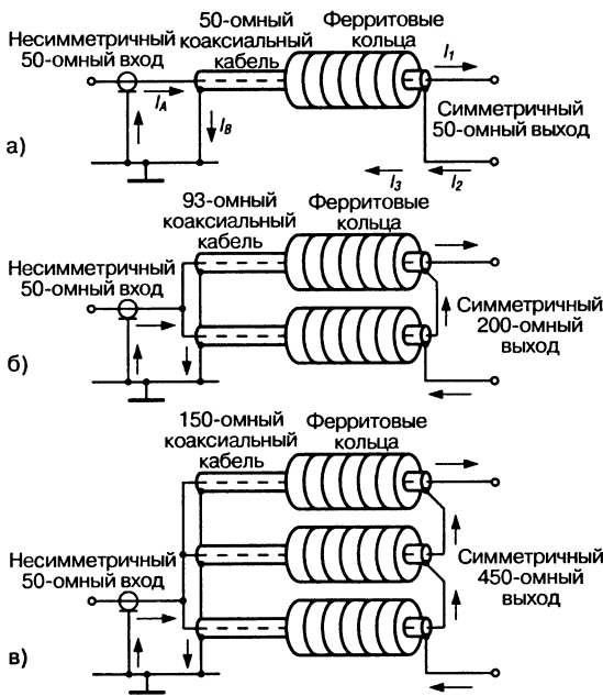
Рис. 7.58. Трансформаторы с коэффициентом преобразования: а – 1:1, б – 1:4, в – 1:9
