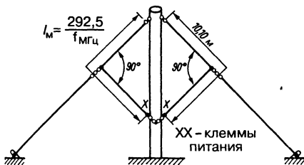
Рис. 13.18. Двусторонний квадрат
