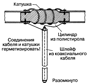
Рис. 18.14. Вариант исполнения средней части рефлектора и директора
