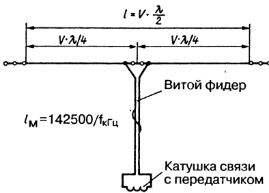
Рис. 10.3. Вибратор с витым фидером
