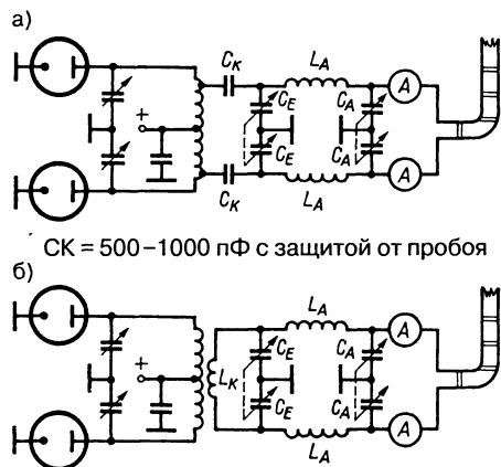
Рис. 8.12. Симметричный П-образный фильтр для антенн с настроенным фидером:
