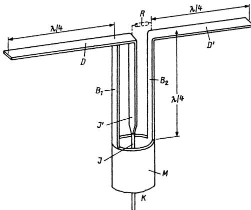
Рис. 7.29. Открытый симметрирующий шлейф
