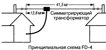
Принципиальная схема FD-4 Рис. 10.16. Многодиапазонная антенна Виндома с питанием по коаксиальному кабелю типа FD4
