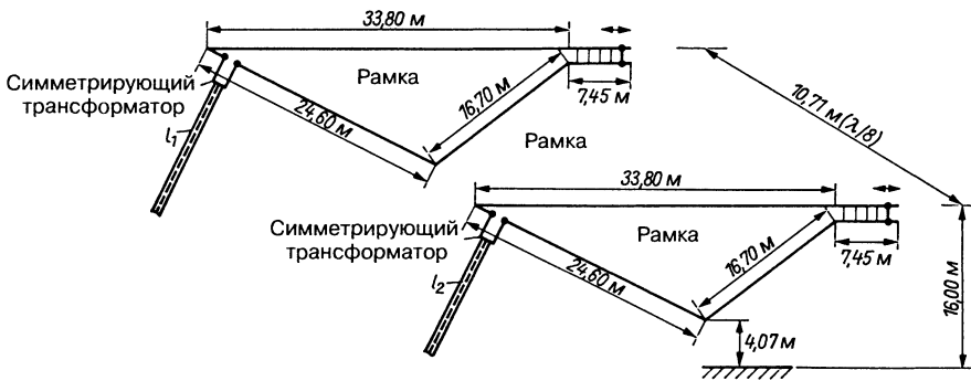
Рис. 19.83. Параметры «монстра» по данным DL6WD
