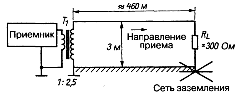
Рис. 12.3. Простая антенна Бевереджа для диапазона 160 м (согласно W8NHS)
