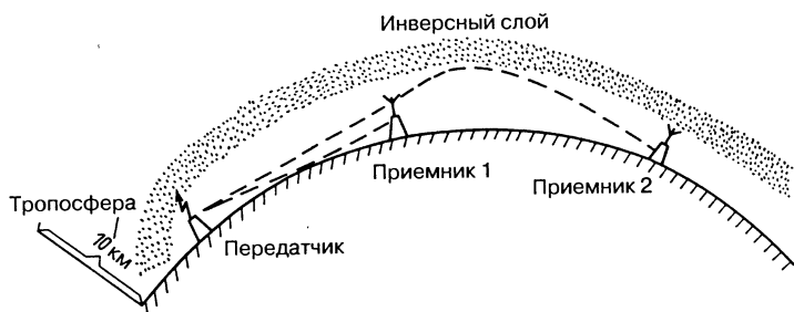
Рис. 2.9. Распространение метровых волн в тропосфере
