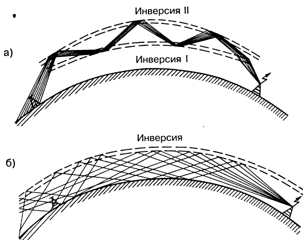
Рис. 2.10. Передача сигнала по тропосферному волноводу
