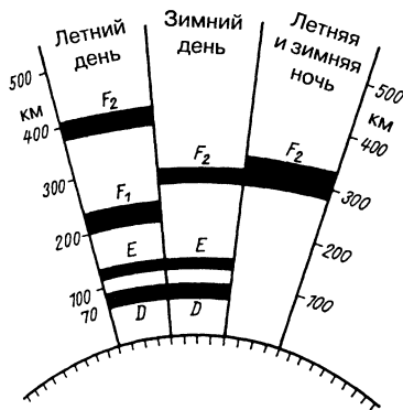
Рис. 2.2. Слои ионосферы
