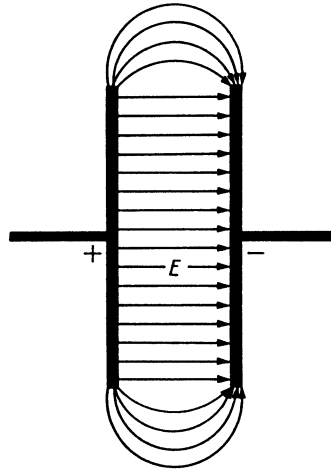
Рис. 1.2. Электрическое поле конденсатора
