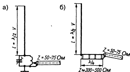
Рис. 19.36. Возбуждение вертикального полуволнового излучателя через коаксиальный кабель
