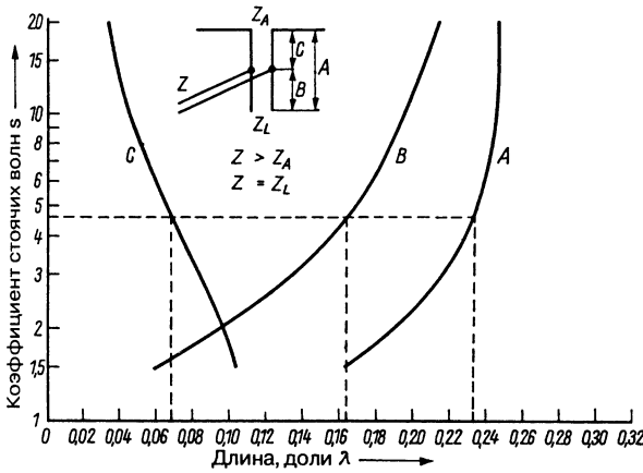
Рис. 6.14. Зависимость длин разомкнутого шлейфа
