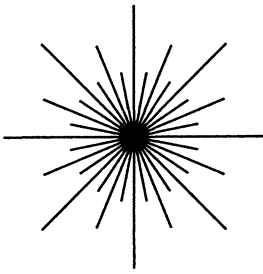
Рис. 19.2. Сеть заземления короткой вертикальной антенны
