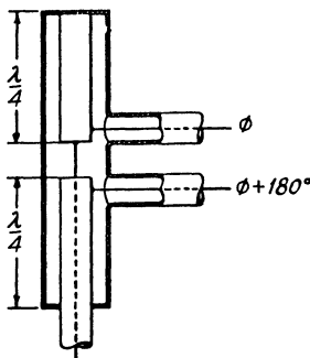
Рис. 7.35. Полуволновый симметрирующий объемный контур
