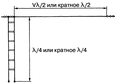
Рис. 10.6. Антенна типа «Цеппелин»
