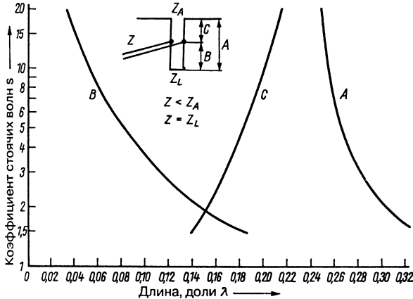
Рис. 6.15. Зависимость длин короткозамкнутого шлейфа
