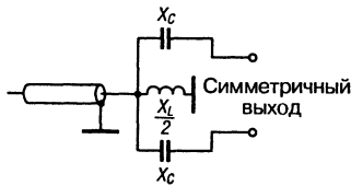
Рис. 7.63. Схема X/2
