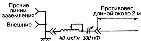
Рис. 11.7. Настроенный противовес в качестве «искусственной земли»
