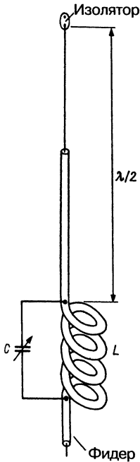
Рис. 7.43. Настроенный контур (контур T 2 LT)
