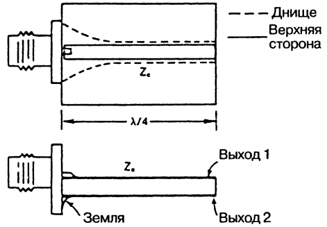
Рис. 7.68. Микрополосковый вариант клинообразного трансформатора
