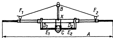
Рис. 18.21. Пассивный элемент антенны DL1FK
