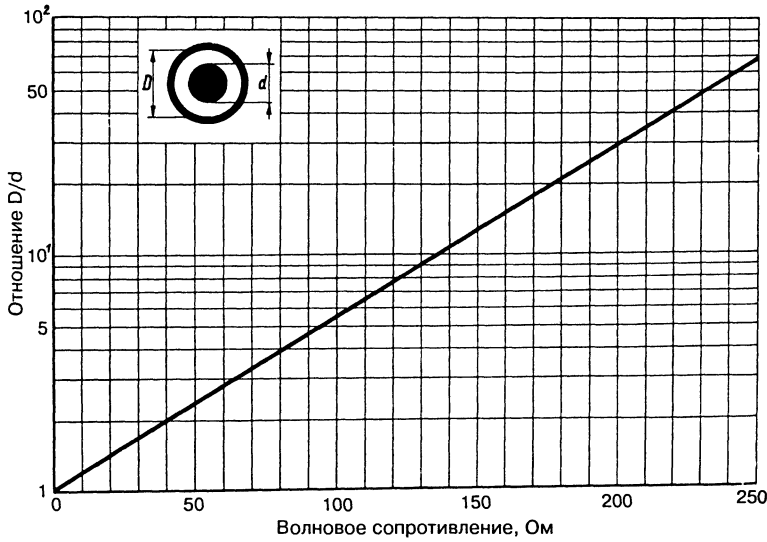
Рис. 5.5. Волновое сопротивление коаксиальной линии с воздушной изоляцией
