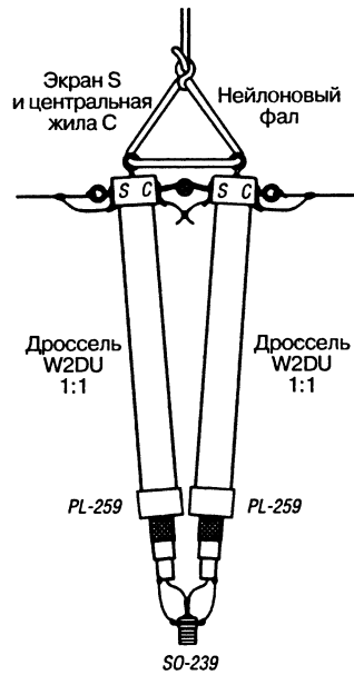
Рис. 7.59. Эскиз трансформатора с коэффициентом 1:4
