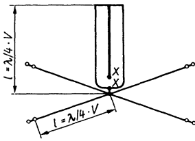
Рис. 19.21. Антенна Groundplane с тремя проводниками
