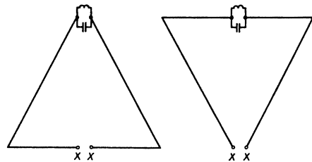
Рис. 15.8. Двухдиапазонный дельтообразный элемент
