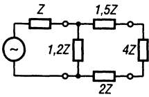
Рис. 7.62. Симметрирующий трансформатор 1:4 на резисторах
