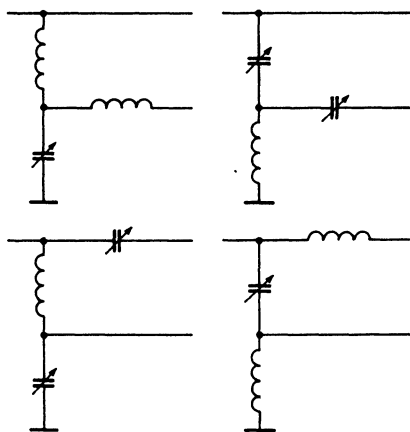
Рис. 7.34. Схема Алфорда
