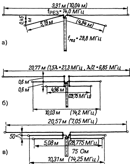
Рис. 10.20. Блок вибраторов: а – влияние межвибраторной связи на резонансную частоту; б – четырехдиапазонная антенна с блоком вибраторов G3ESP; в – четырехдиапазонная антенна с блоком вибраторов G14JTF
