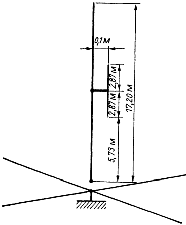
Рис. 19.63. Вертикальная антенна W1JF для диапазонов 30 и 12 м
