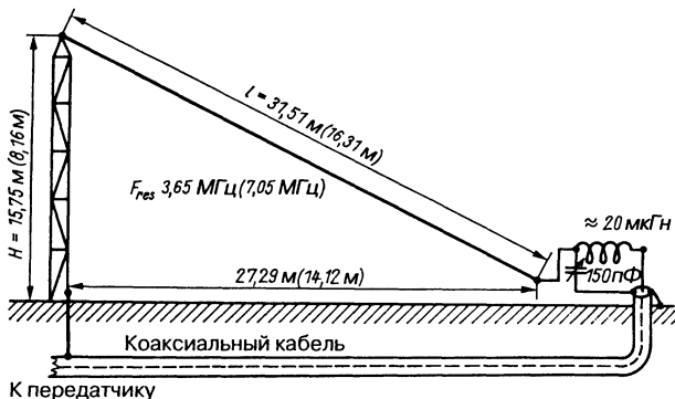
Рис. 19.78. Практическое исполнение половинчатой антенны Delta-Loop для диапазона 80 м (числа в скобках приведены для 40-метрового диапазона)
