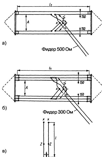
Рис. 14.7. Антенны W8JK с петлевыми элементами: а – с простыми петлевыми вибраторами и линиями l_2 из плоского 240-омного кабеля; б – с двойными петлевыми вибраторами и линиями l_2 из плоского 300-омного кабеля; в – шлейф к версиям а и б
