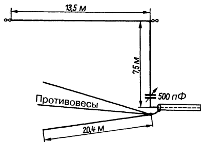
Рис. 19.40. Г-образная антенна для 3,5 МГц
