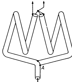
Рис. 7.25. Расположение витков широкополосного симметрирующего шлейфа
