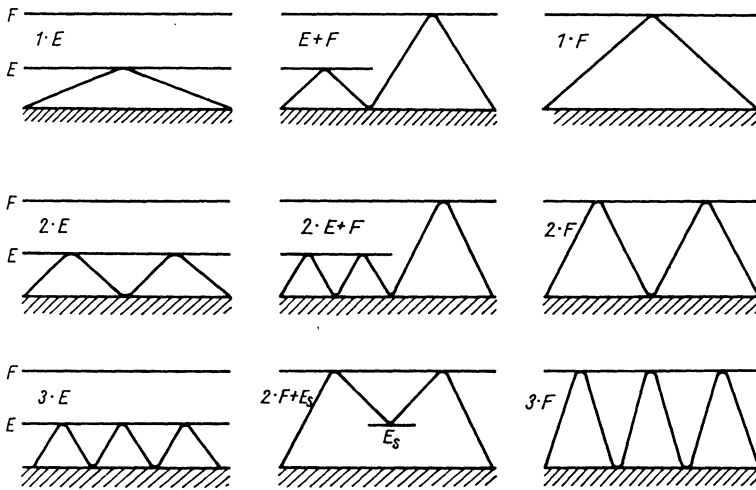
Рис. 2.5. Схематическое изображение некоторых ионосферных отражений радиоволн
