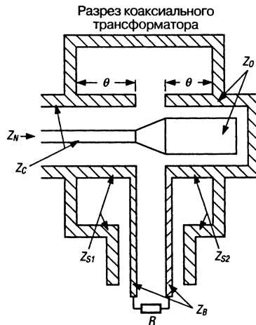
Рис. 7.39. Коаксиальное исполнение скомпенсированного симметрирующего трансформатора в разрезе
