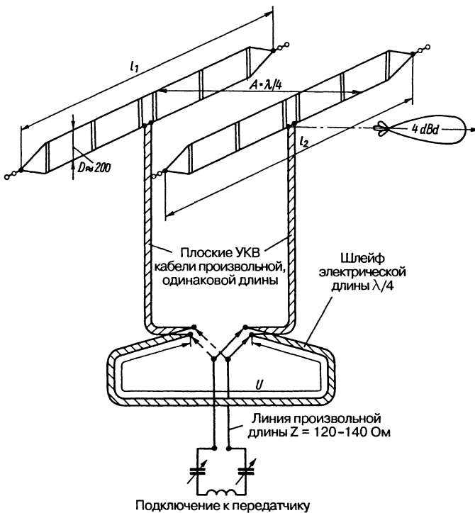
Рис. 14.14. Двухэлементный направленный излучатель с электрически переключаемой ориентацией главного луча
