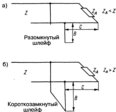
Рис. 6.13. Схема согласующего шлейфа:
