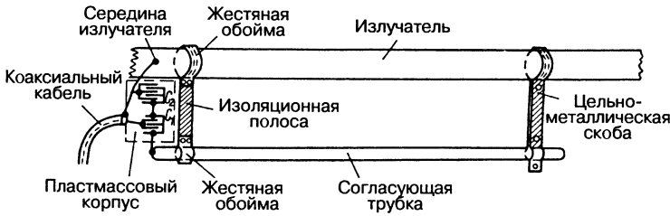
Рис. 6.7. Рекомендуемое устройство согласующего звена
