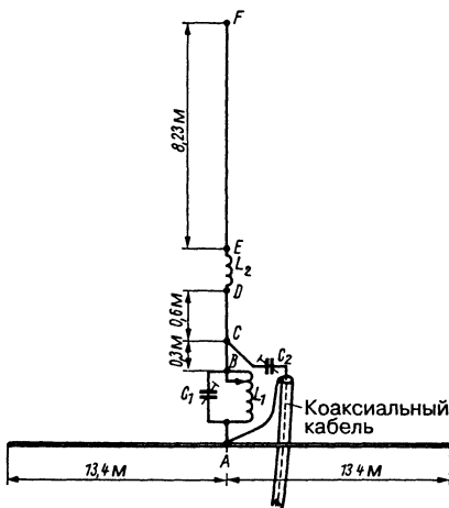
Рис 19.60 Схема двухдиапазонной Groundplane для 80- и 40-метрового диапазонов
