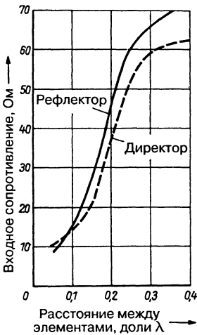
Рис. 16.5. Зависимость входного сопротивления антенны от расстояния между полуволновым вибратором и пассивными элементами
