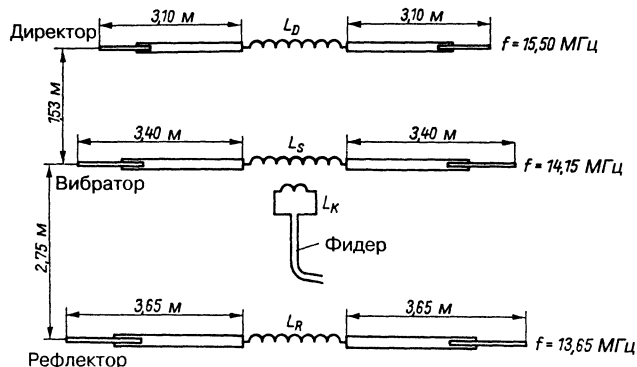
Рис. 17.2. Трехэлементная миниатюрная остронаправленная антенна 20-метрового диапазона VK2AOU
