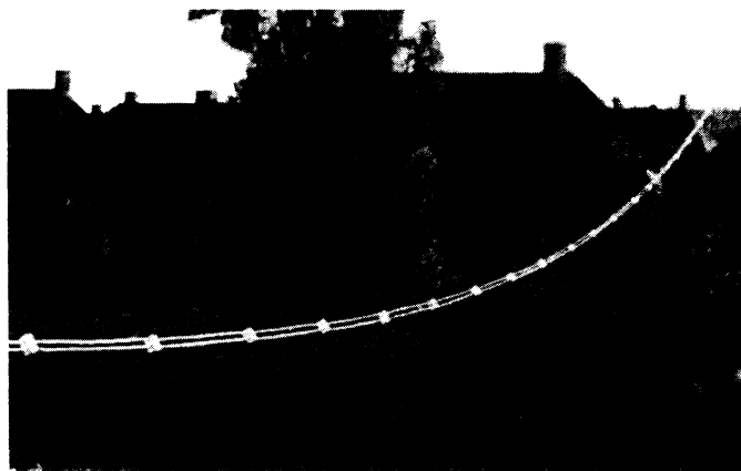
Рис. 5.31. Фидер с волновым сопротивлением 300 Ом
