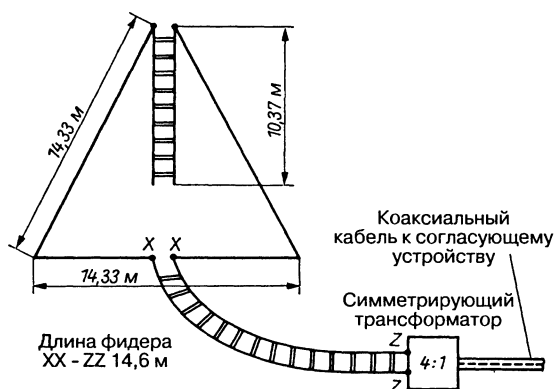
Рис. 15.9. Многодиапазонная дельтообразная антенна
