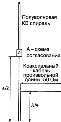
Рис. 19.86. Спиральная КВ антенна с подводкой кабеля
