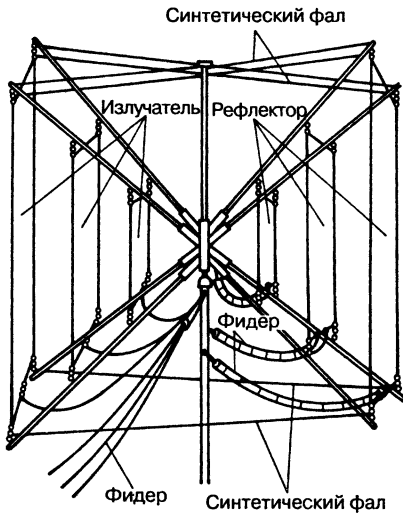
Рис. 18.45. Трехдиапазонная двойная рамочная антенна
