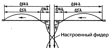
Рис. 11.19. Распределение тока в удлиненном двойном «Цепелине»
