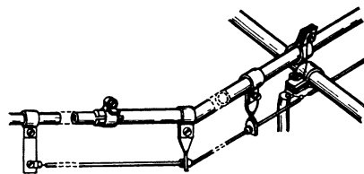
Рис. 15.22. Конструкция гамма-согласователя
