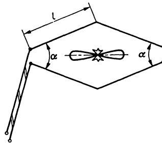
Рис. 11.18. Двунаправленная ромбическая антенна
