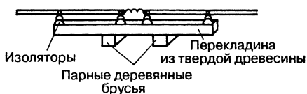
Рис. 18.13. Вариант крепления элементов антенны G4ZU
