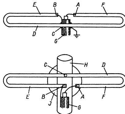
Рис. 7.45. Интегральный симметрирующий трансформатор
