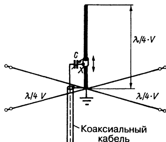
Рис 19.17. Вариант заземления антенны Groundplane
