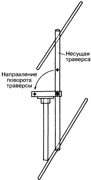
Рис. 16.14. Крепление направленного излучателя на трубе мачты
