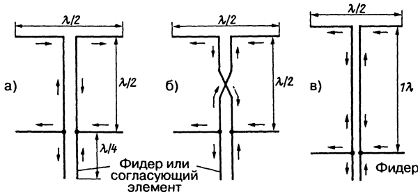
Рис. 13.6. Возбуждение двух параллельных вибраторов
