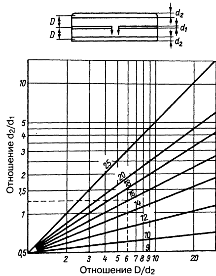
Рис. 3.25. Коэффициент кратности двойного петлевого вибратора
