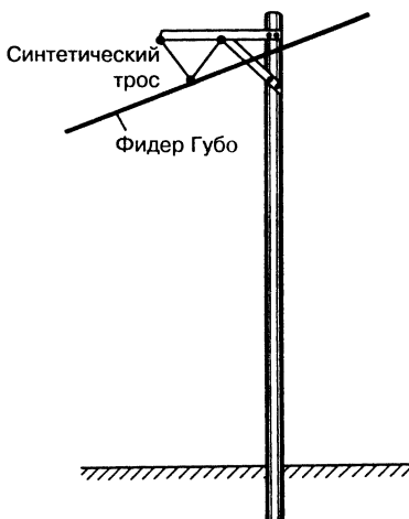
Рис. 5.17. Рациональное крепление фидера Губо
