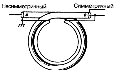
Рис. 7.50. Кабельный дроссель с добавочным витком
