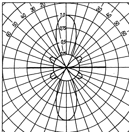
Рис. 11.20. Идеализированная диаграмма направленности в плоскости E
