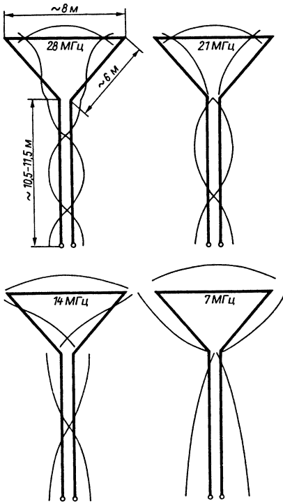
Рис. 18.35. Схема и распределение тока многодиапазонной дельтаобразной антенны НВ9АDQ
