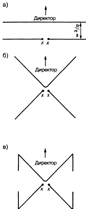
Рис. 16.15. Формирование X-образного направленного излучателя
