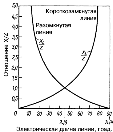
Рис. 5.30. Графики для определения реактивных сопротивлений
