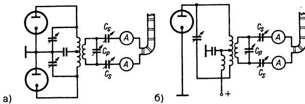
Рис. 8.10. Подключение настроенного фидера: а – к двухтактному оконечному каскаду, б – к однотактному оконечному каскаду
