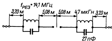
Рис. 10.26. Модификация антенны W3DZZ для трех диапазонов
