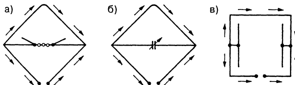
Рис 17.8 Схемы укороченных рамочных элементов
