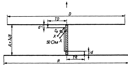
Рис. 14.13. Размеры антенны HB9CV
