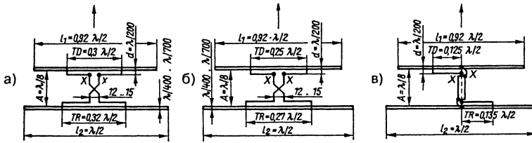
Рис. 14.12. Устройство и размеры остронаправленной антенны HB9CV с разным входным сопротивлением: а – 300 Ом; б – 150 Ом; в – 75 Ом
