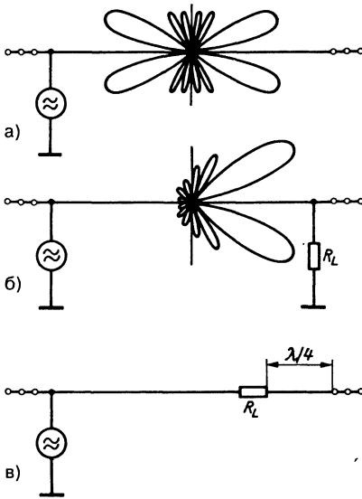
Рис. 12.2. Сравнение идеализированных горизонтальных диаграмм направленности: а – согласованная длинноволновая антенна длиной 3\lambda ; б – замкнутая антенна той же длины; в – замкнутая антенна с противовесом длиной \lambda/4
