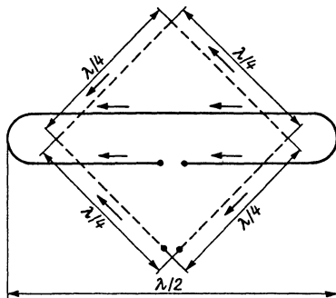
Рис. 15.1. Превращение петлевого вибратора в квадратный элемент
