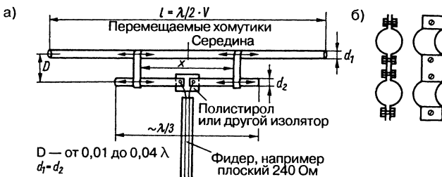
Рис. 6.2. Согласующий Т-трансформатор: а – рекомендуемая компоновка; б – зажимные скобы
