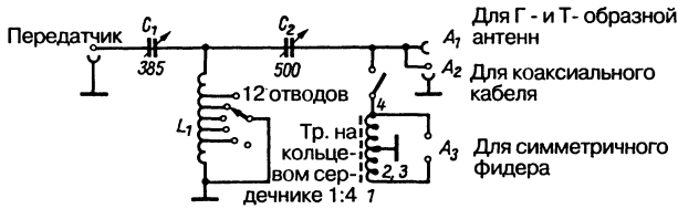
Рис. 8.16. Т-образный СЛП
