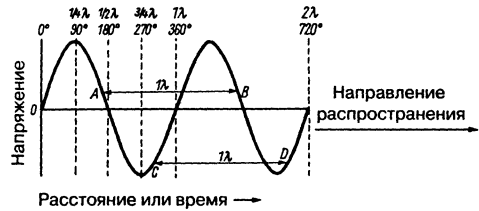
Рис. 1.1. График электромагнитной волны
