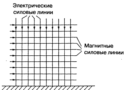
Рис. 1.5. Плоский волновой фронт с вертикальной поляризацией
