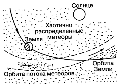
Рис. 2.12. Орбиты Земли и потока метеоритов
