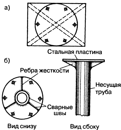
Рис. 18.49. Крепление перекрестия на мачте: а – опорная пластина; б – металлический фланец после сварки
