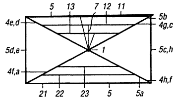
Рис. 18.64. Антенна Low Base Quad, вид сверху
