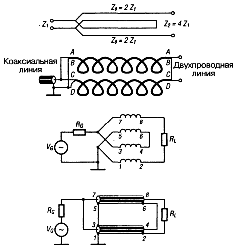
Рис. 7.8. Преобразование сопротивления в пропорции 1:4
