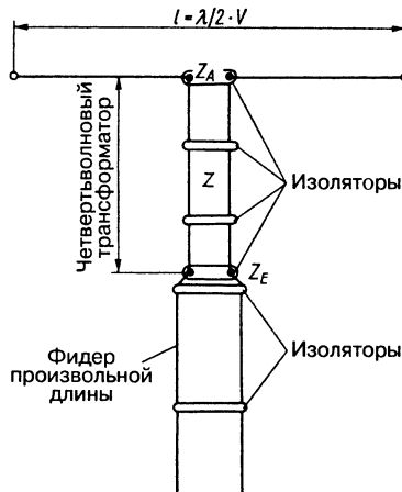
Рис. 6.8. Четвертьволновый трансформатор
