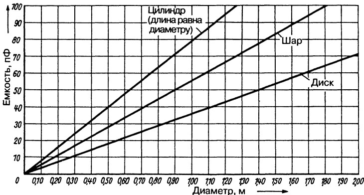
Рис. 19.32. Зависимость емкости диска, шара и цилиндра от диаметра d
