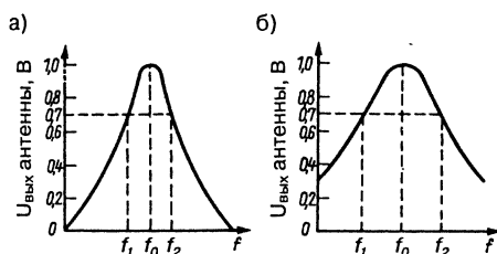
Рис. 3.5. Резонансная кривая излучателя и ширина полосы B = f_2 - f_1 ; а – при большом, б – при малом отношении L/C
