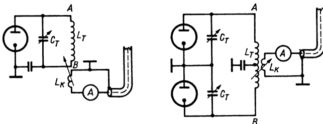
Рис. 8.2. Улучшенный способ подключения коаксиального кабеля
