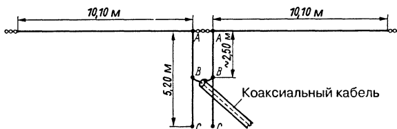
Рис. 10.18. Трехдиапазонный вибратор
