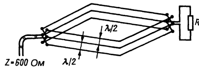
Рис. 12.13. Ромбическая антенна с поэтажным расположением излучателей
