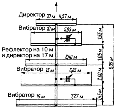
Рис. 18.40. Двухдиапазонная остронаправленная антенна W4KFC с вложенными элементами на 10 и 15 м
