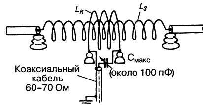
Рис. 17.3 Усовершенствованное индуктивное согласование
