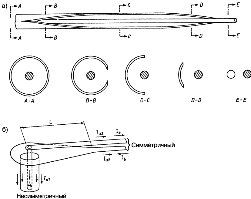
Рис. 7.67. Коаксиальный вариант клинообразного трансформатора
