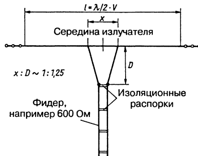
Рис. 6.1. Согласующий дельта-трансформатор
