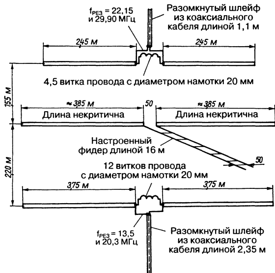
Рис. 18.12. Модификация антенны G4ZU
