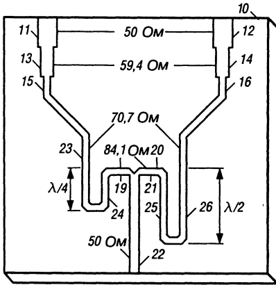
Рис. 7.16. Реактивный симметрирующий трансформатор
