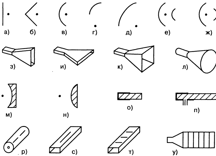
Рис. 4.4. Апертурные излучатели: а – плоское зеркало; б – уголкового отражатель; в – осесимметричная параболическая антенна; г – параболический рупор (вырезка параболоида с рупорным облучателем); д – офсетная параболическая антенна; е – антенна Кассегрена; ж – антенна Грегори; з – E-плоскостной секториальный рупор; и – H-плоскостной секториальный рупор; к – пирамидальный рупор, л – конический рупор; м – ускоряющая линза; н – замедляющая линза; о – линза ближнего поля; п – полистироловая стержневая антенна; р – щелевая антенна коаксиальной линии; с, т – волноводные щелевые антенны; у – гофрированная антенна
