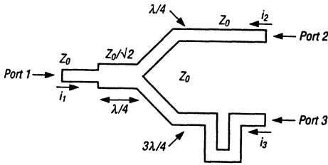
Рис. 7.15. Реактивный симметрирующий трансформатор
