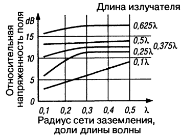
Рис. 19.5. Зависимость относительной напряженности поля от радиуса сети заземления для вертикальных излучателей разной длины
