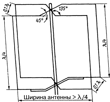
Рис. 15.17. Схема антенны «швейцарский квадрат»
